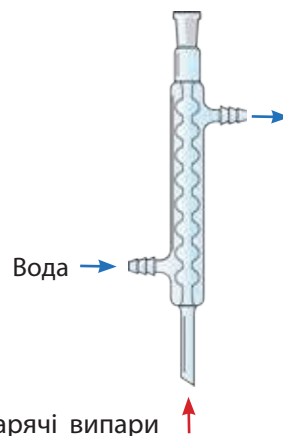
Мал. 2. Кульковий обернений холодильник Алліна
